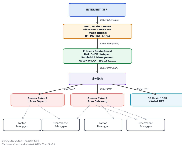
Gambar 2.1 Rancangan Simulasi Jaringan untuk Cisco Packet Tracer
